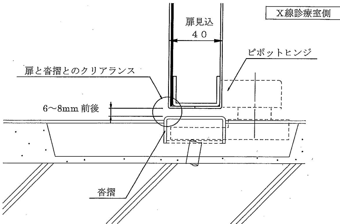
鋼製扉と沓摺のクリアランス
