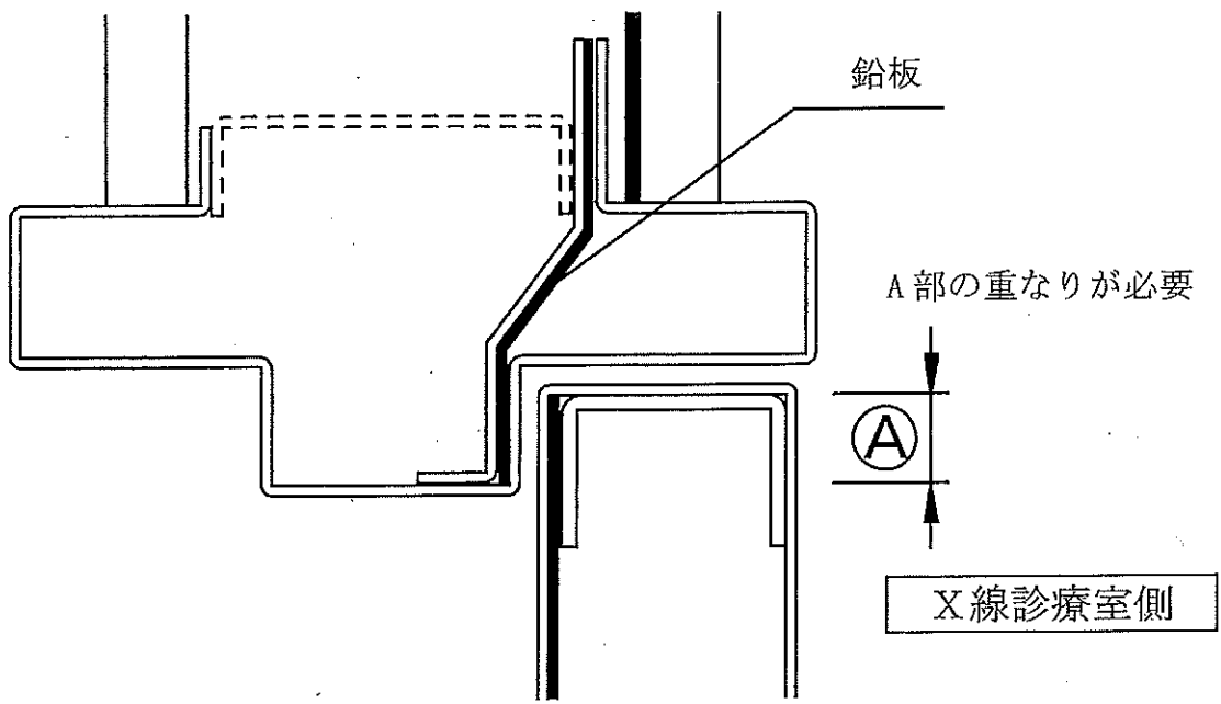
鋼製防護建具詳細
