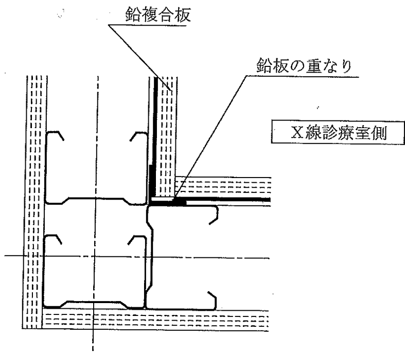
画壁 鉛複合板入隅部詳細
