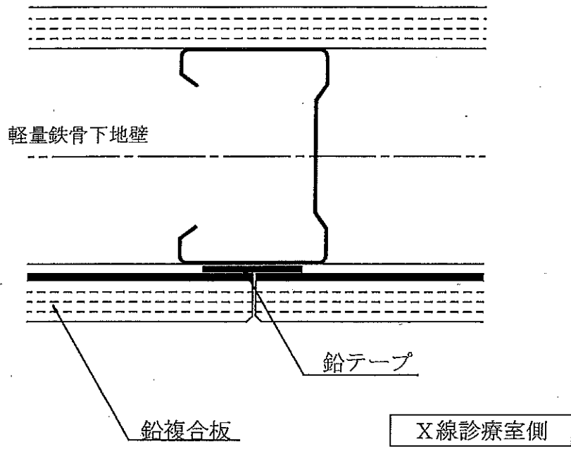
鉛複合板の接合部詳細
