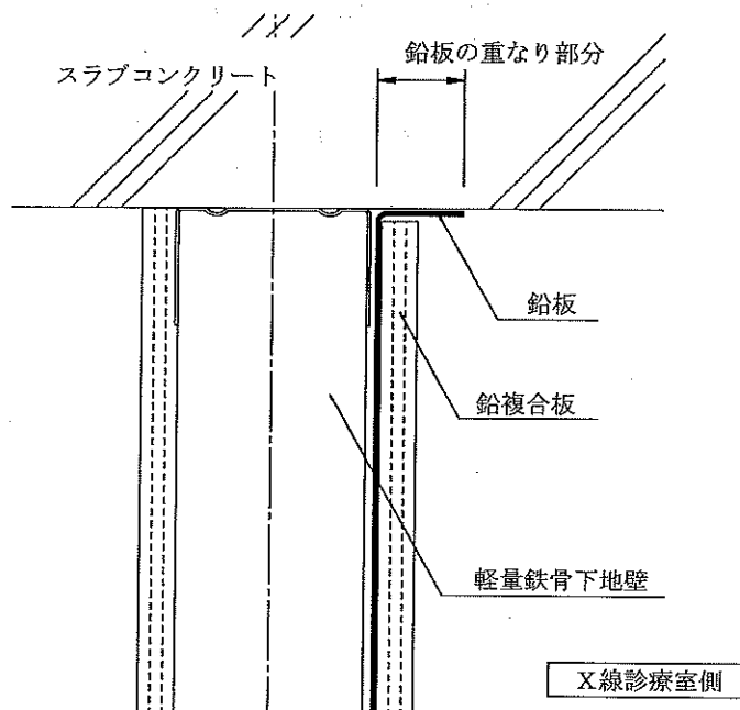
鉛複合板端部詳細
