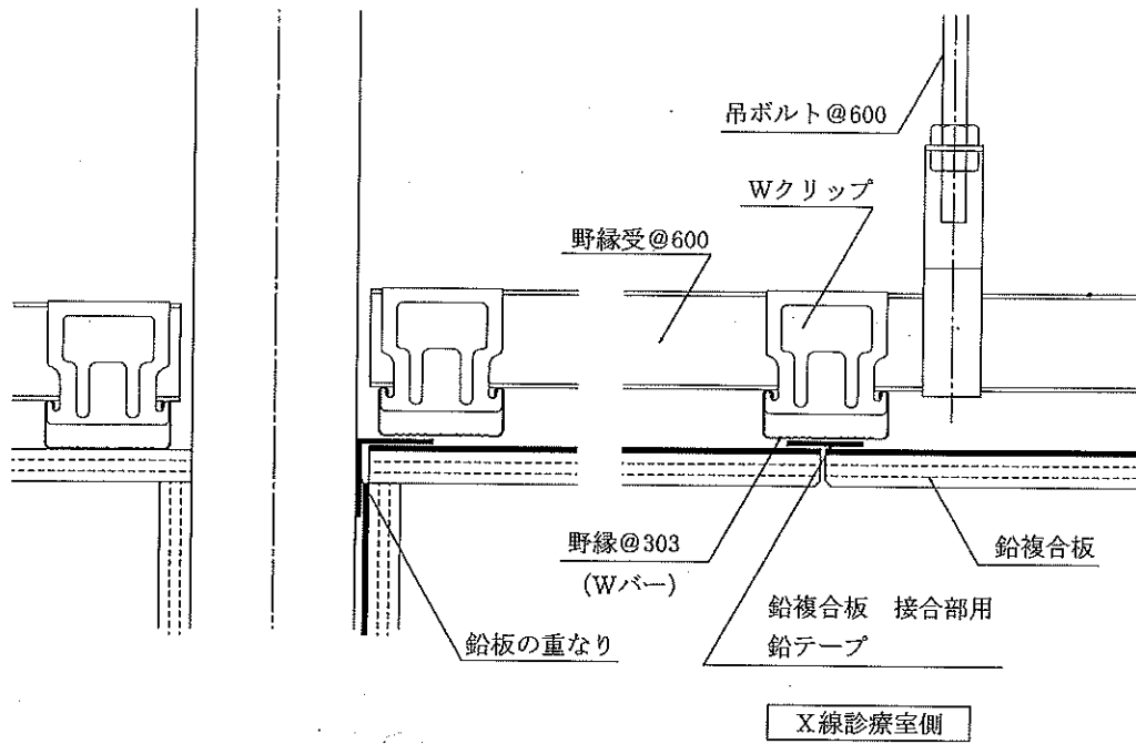
鉛複合板天井面詳細
