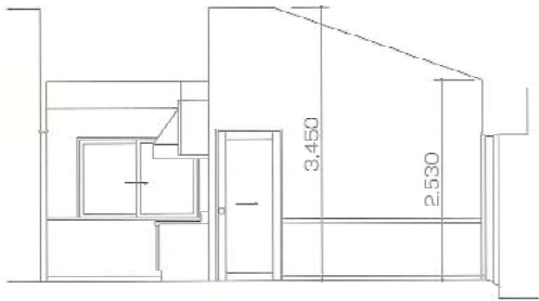
a-a断面図 1007
