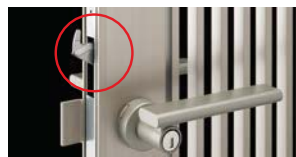
鎌錠(シリンダーPA錠)
