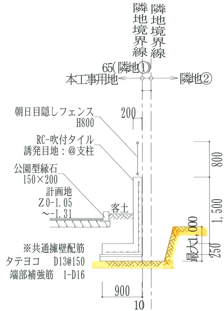
理想な掘削方法
