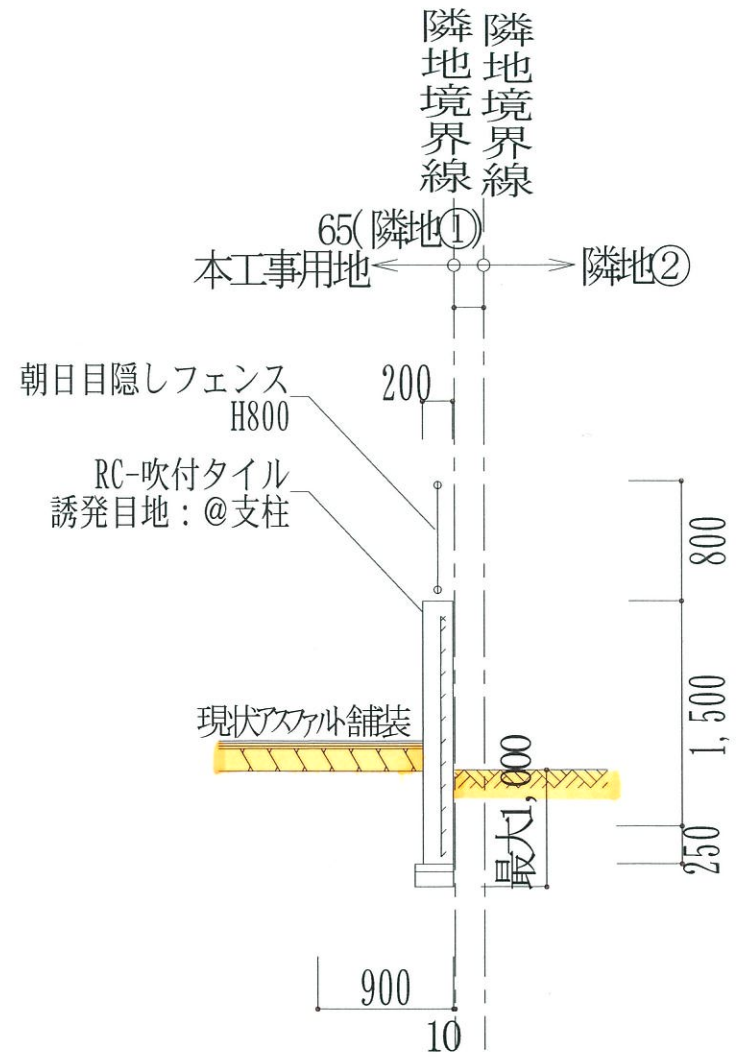
現況擁壁詳細図
