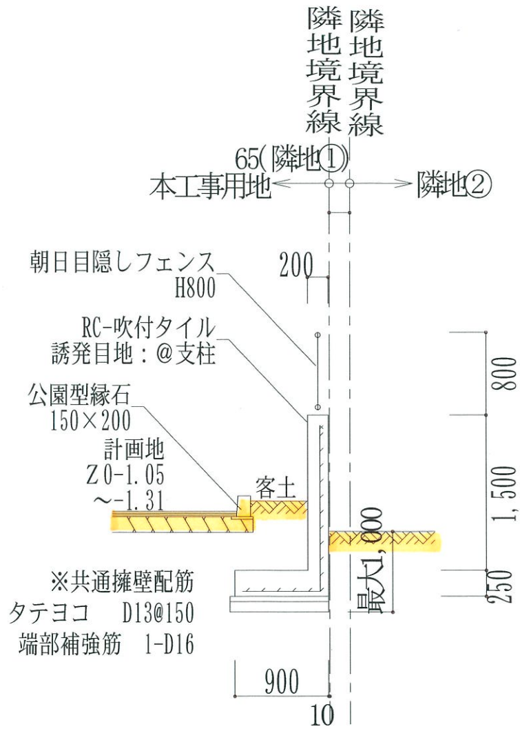
計画擁壁詳細図
