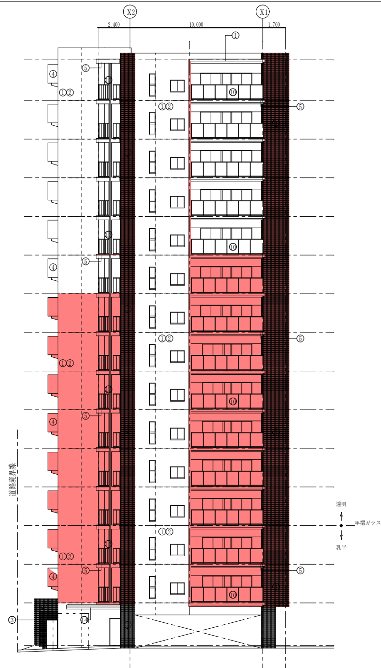
北側立面図
