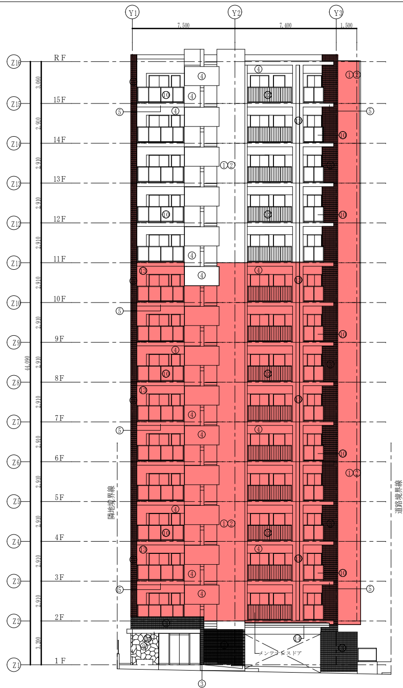
東側立面図
