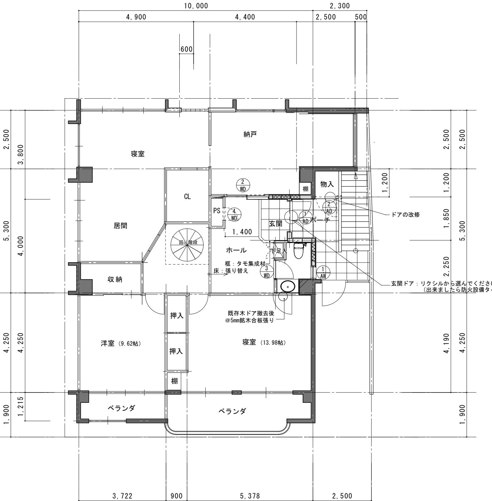
(改修後) 平面図S=1/100
